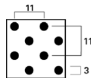
Perfo 4 (Lochanteil 11,7%)
